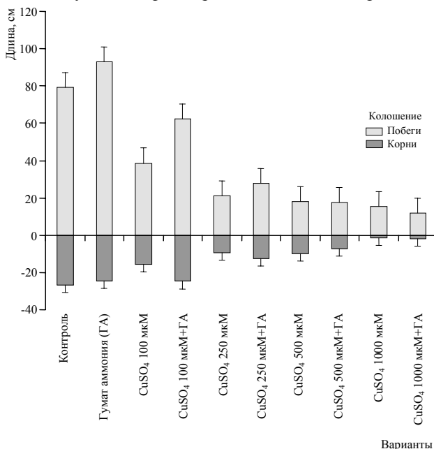
Рис. 1. Влияние высоких концентраций меди и гумата на линейный рост растений пшеницы; бары на диаграмме показывают значения НСР 05
